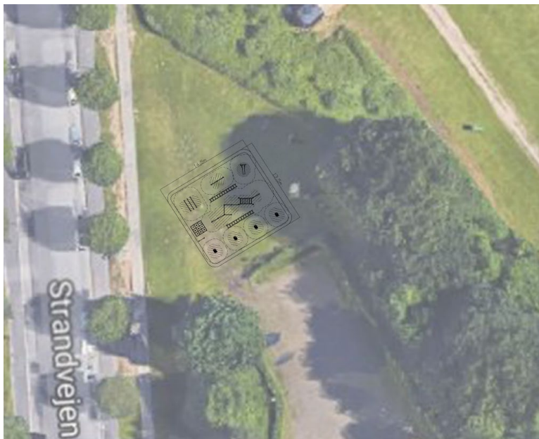
Figur 2 Situationsplan over placering af fitnessområde hvor bunden etableres med faldunderlag
