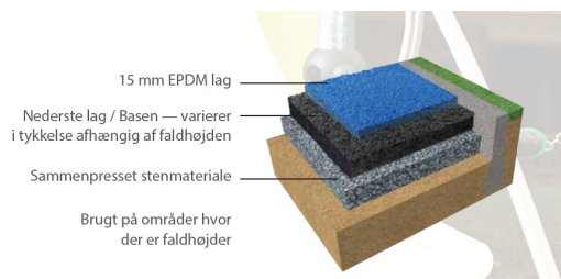
Figur 4. Underlaget ved fitnessområdet består af FLEXOTOP TM
