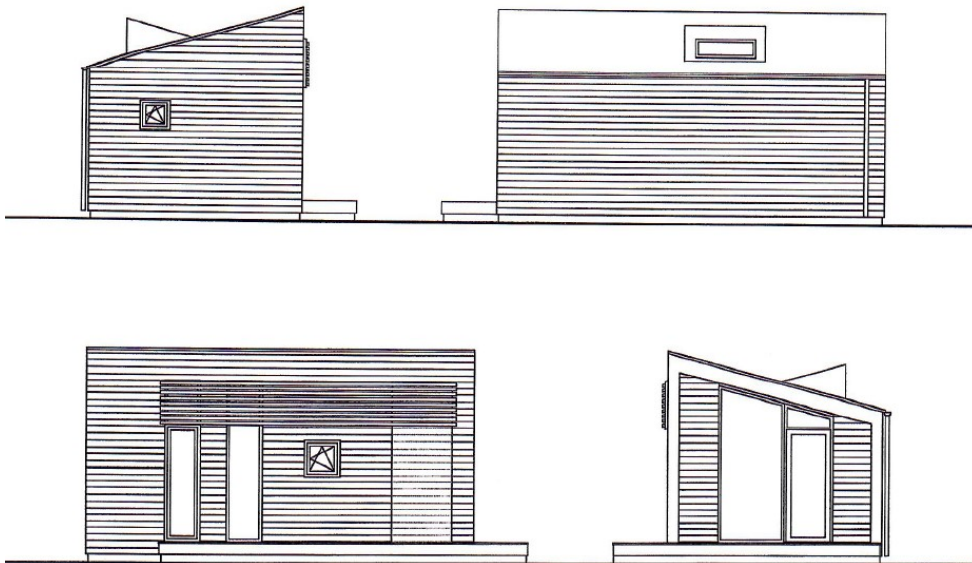
Tegning af facaderne på de ansøgte campinghytter
