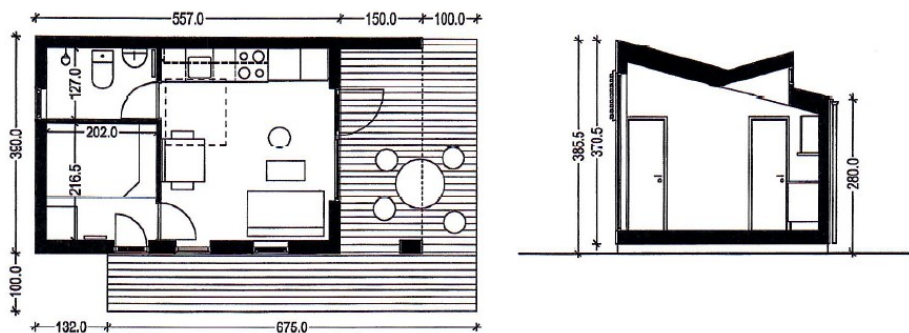
Grundplan og snit af hytterne.
