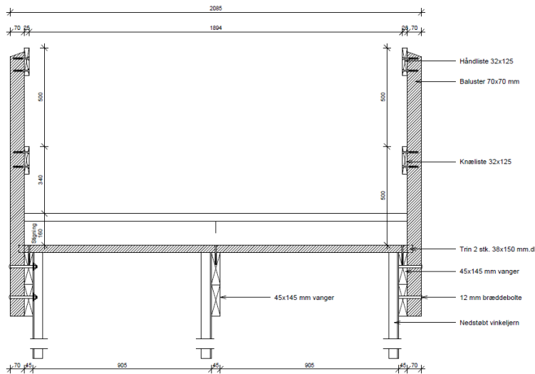
Tværsnit trappe
