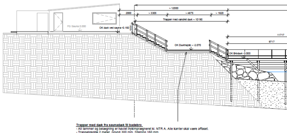
Tværsnit af anlægget
