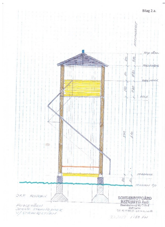
Bilag fra ansøgning, tegning af fugletårn
