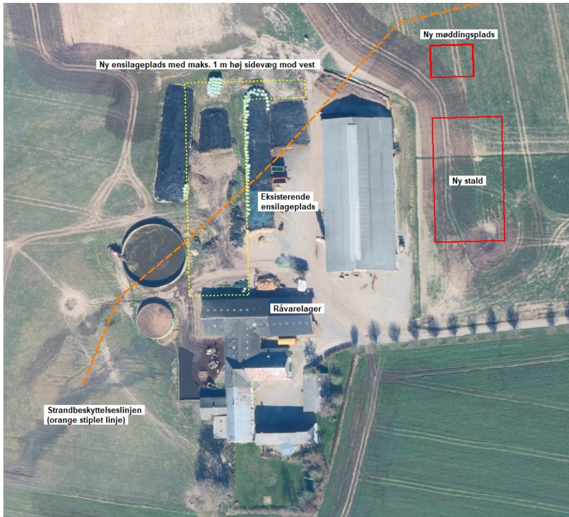
Figur 1. Situationsplan viser eksisterende og planlagte anlæg. Strandbeskyttelseslinjen er vist med orange streg, og de strandbeskyttede arealer ligger nordvest for denne.
