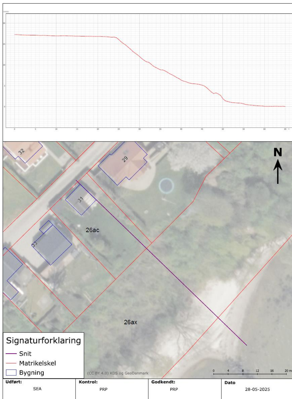
Fig.3. Skitse fra ansøgningen viser det ansøgte snit gennem matriklen til stranden.
