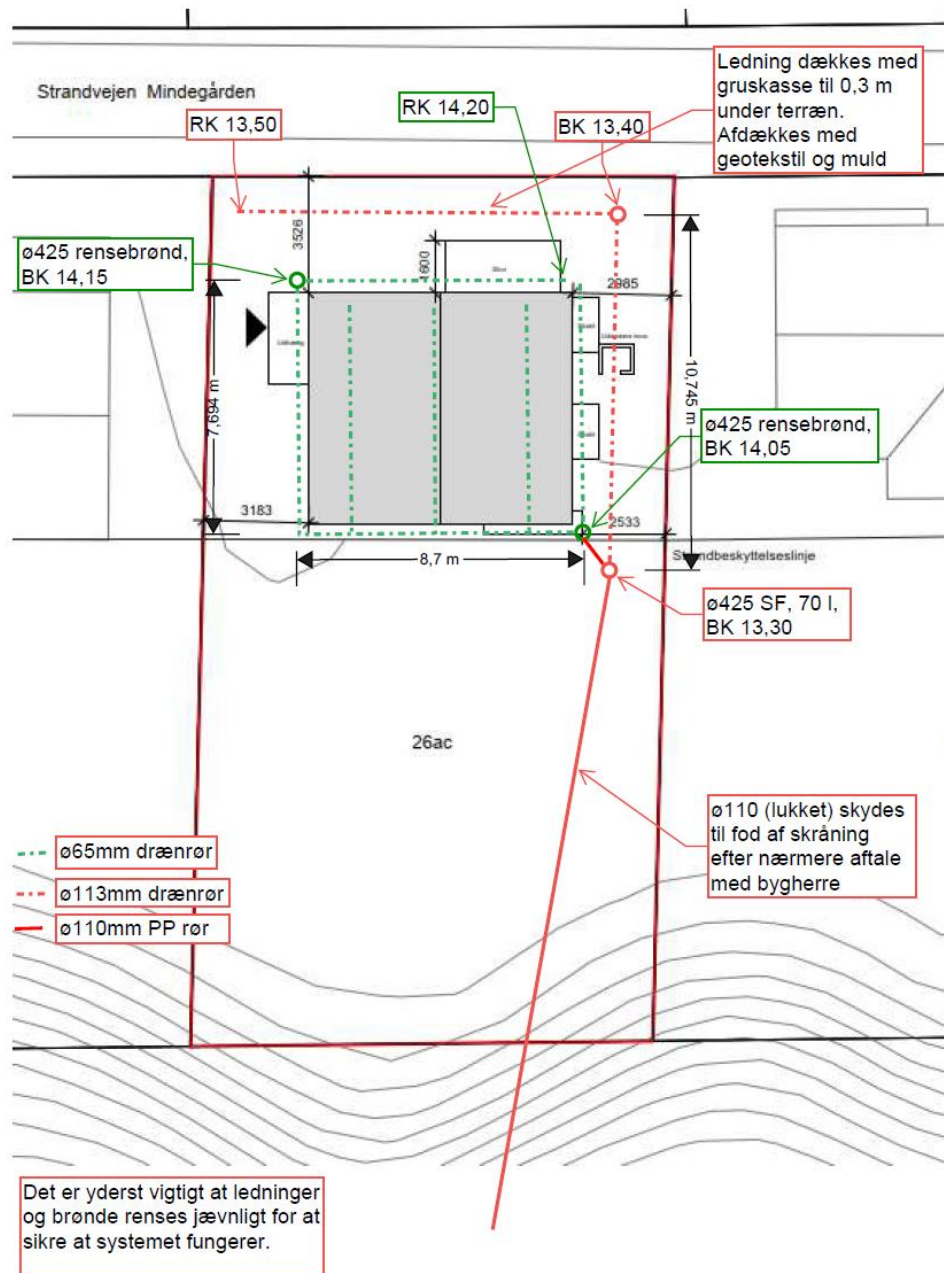
Fig. 2. Skitse fra ansøgningen over rørledning, der ønskes underboret på grunden og ført igennem kystskrænten på matr. 26ax Hejls By, Hejls, til skræntfoden med udløb på stranden.
