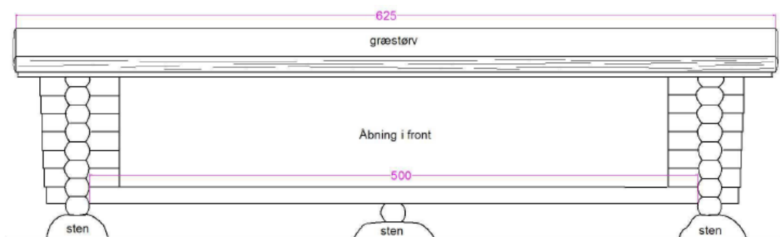
Fig. 3. Tilsendt fra ansøger. Skitse med mål af de ansøgte shelters forfra.
