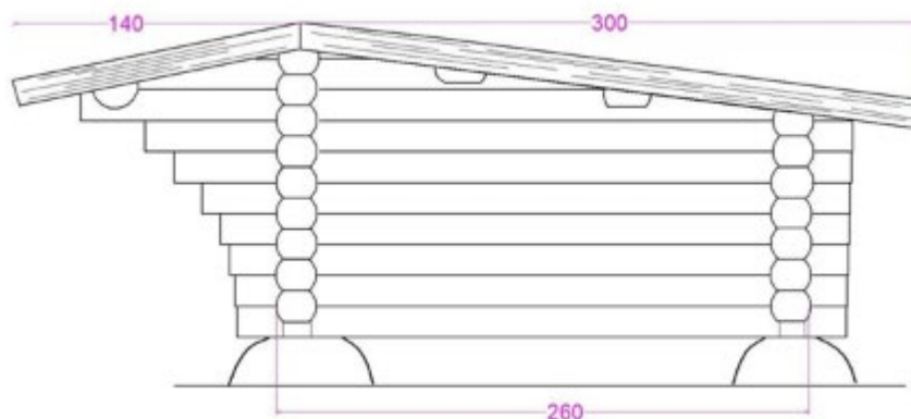
Fig. 4. Tilsendt fra ansøger. Skitse med mål af de ansøgte shelters fra gavlen.
