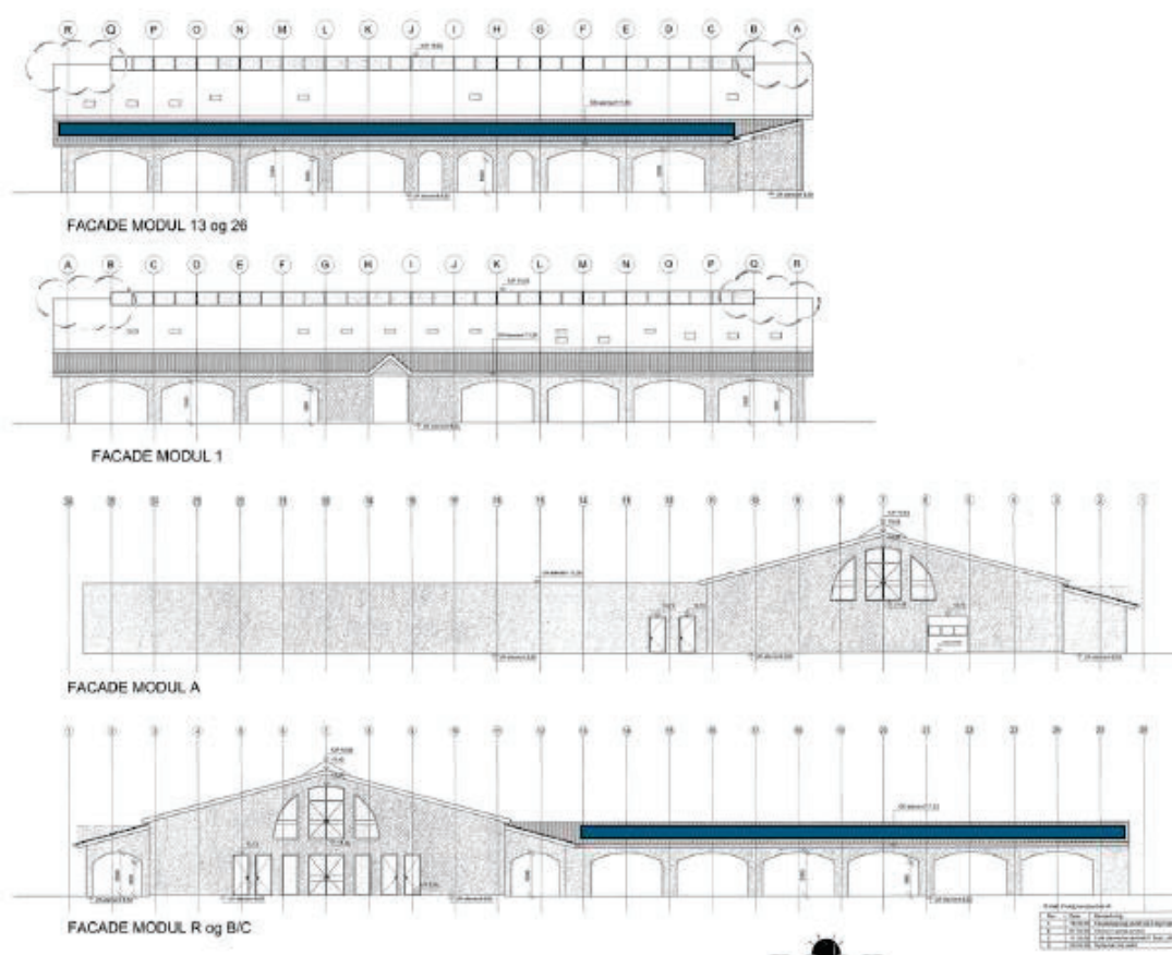
Fig. 4. Tilsendt fra ansøger. Øverste blå markering viser de sydvendte solceller - nederste blå markering viser placering af de vestvendte solceller.
