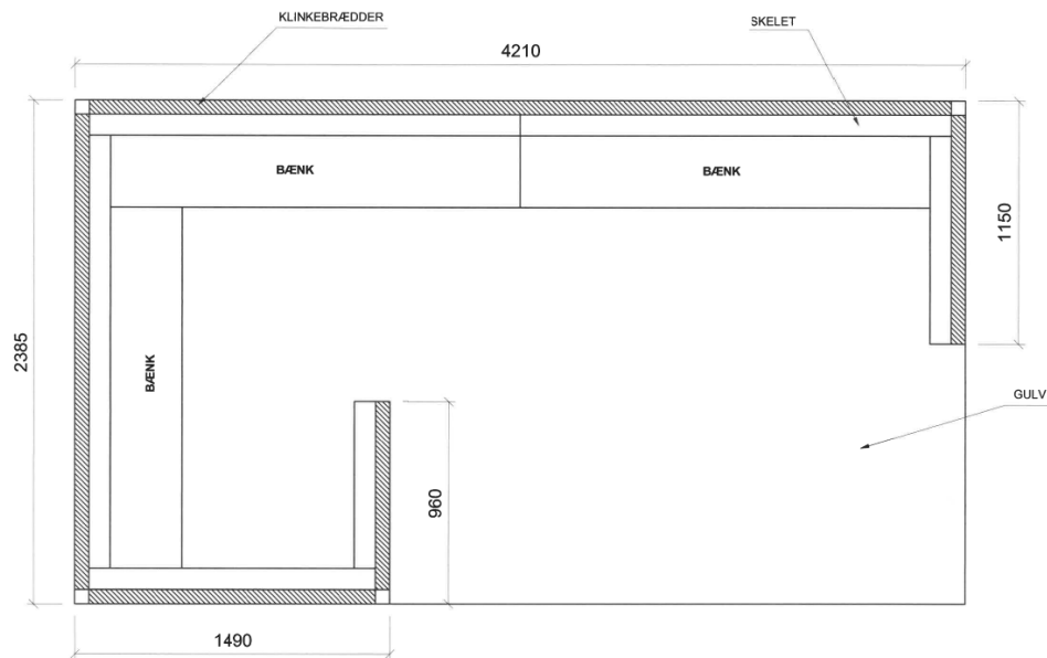
Fig. 4 viser en plantegning over bygningen med mål ovenfra uden tag. Det ses at der opføres siddebænke indvendigt i forbindelse med omklædning. Indsat fra ansøgning.
