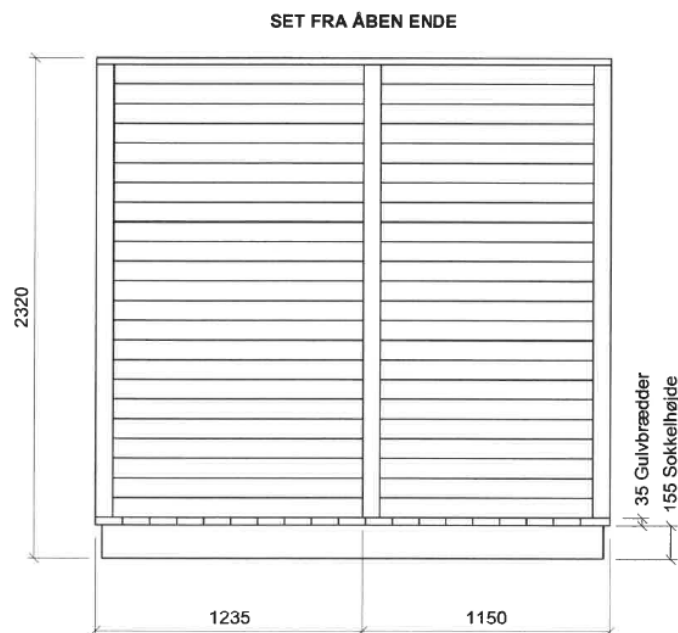
Fig. 5 viser bygningen set fra den åbne ende. Højden på bygningen bliver i alt ca. 2,3 m. Indsat fra ansøgning.
