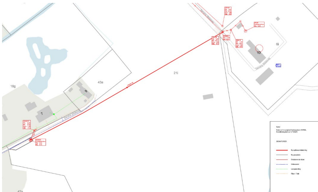
Fig. 2. Tilsendt fra ansøger. Plantegning af den ansøgte pumpestation med elskab markeret med rød prik samt trykledningen markeret med rød linje. Arealet markeret med en boks i venstre nederste hjørne er arealet som ansøges belagt med stabilgrus.
