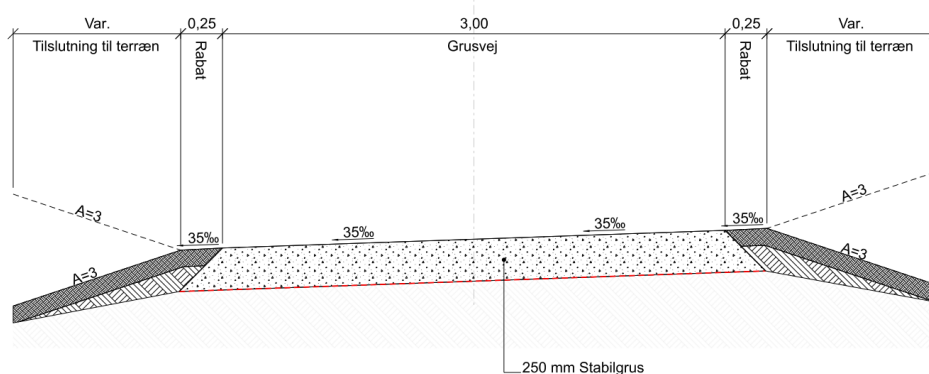
Tværsnit af ny grusvej
