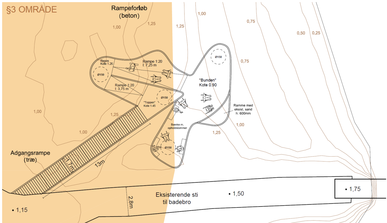
Fig. 4. Tilsendt fra ansøger. På figuren ses en illustration af anlæggets udformning.
