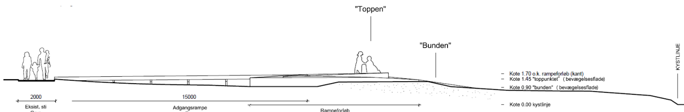
Fig. 5. Tilsendt fra ansøger. Principsnit over anlægget.
