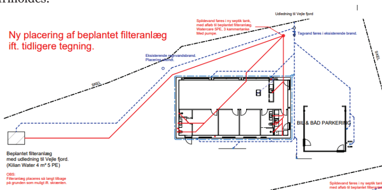
Kloakplan med ny placering
