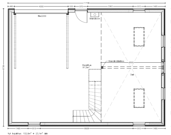
Grundplan – trappen fører op til hems over højre del af huset
