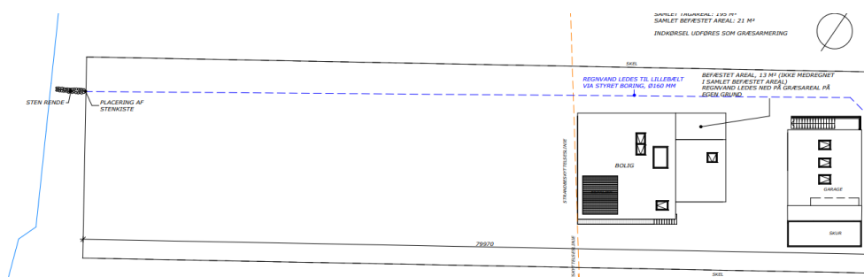
Underboringen og udløbets placering
