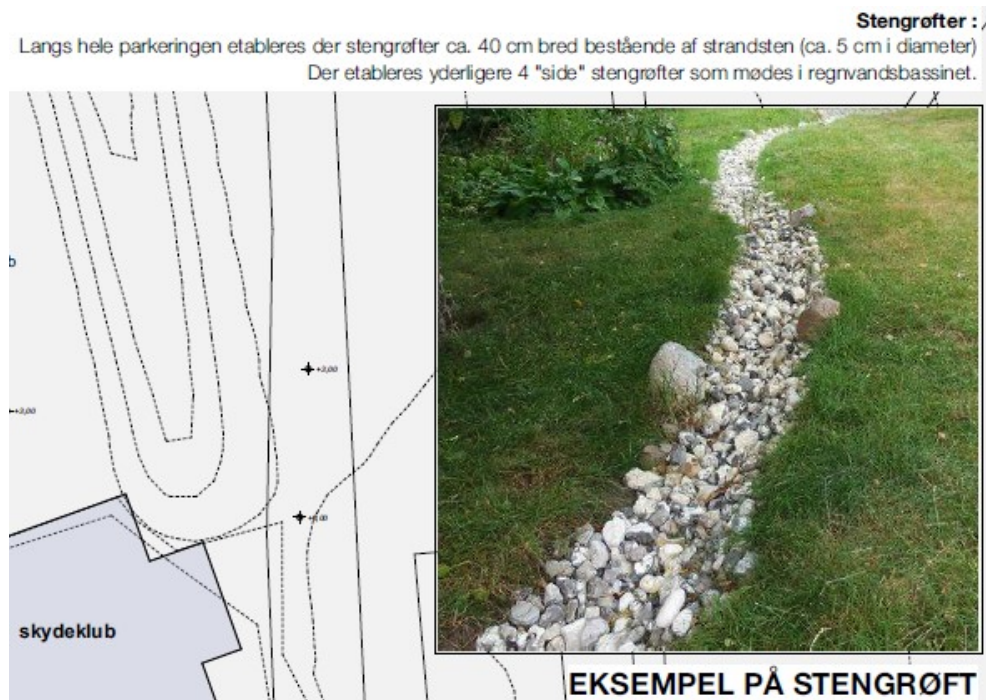
Fig. 5. Tilsendt fra ansøger. Et billede af, hvordan stengrøfterne kommer til at se ud.
