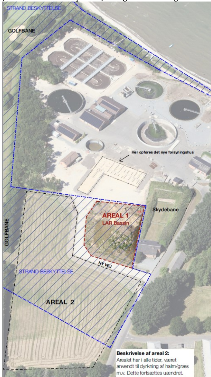
Fig. 2. Tilsendt fra ansøger. Bilag A, der viser den ansøgte placering af LAR bassinet.
