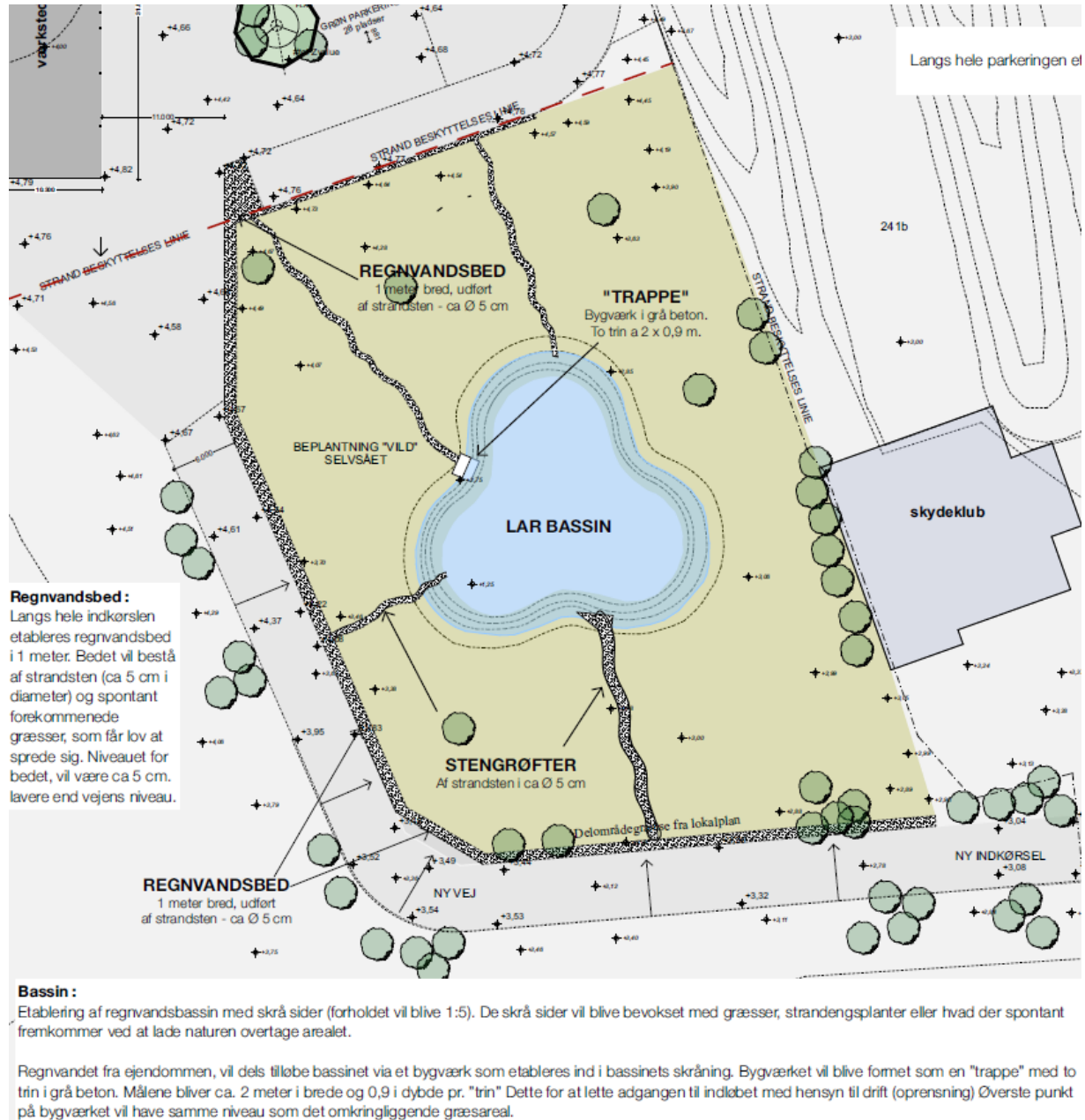
Fig. 3. Tilsendt fra ansøger. Illustration af, hvordan LAR bassin og det omkringliggende areal vil komme til at se ud.
