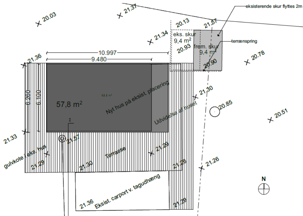
Figur 4: Situationsplanen for det fremtidige sommerhus
