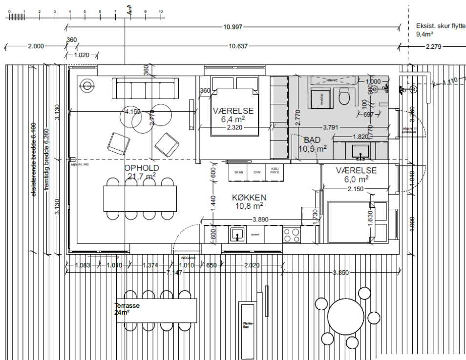
Figur 5: Grundplanen for det fremtidige sommerhus.
