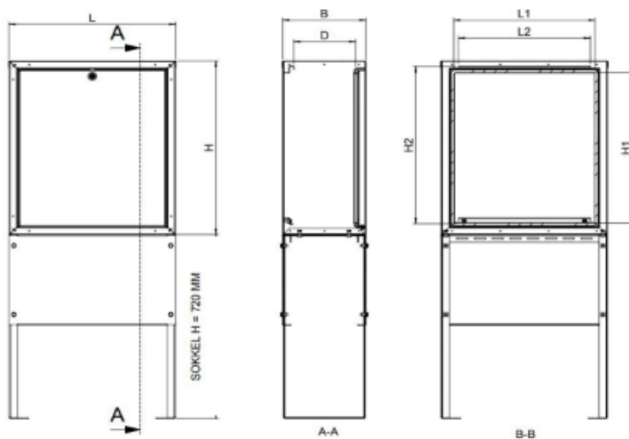
Fig. 3. Tilsendt fra ansøger. Skitsetegning af det ansøgte teknikskab.
