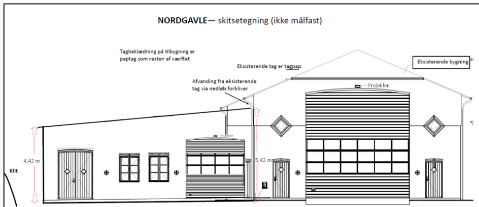
Skitse af gavle mod nord. Til højre ses den eksisterende værftsbygning. Til venstre ses den lavere tilbygning med ensidig taghældning.
