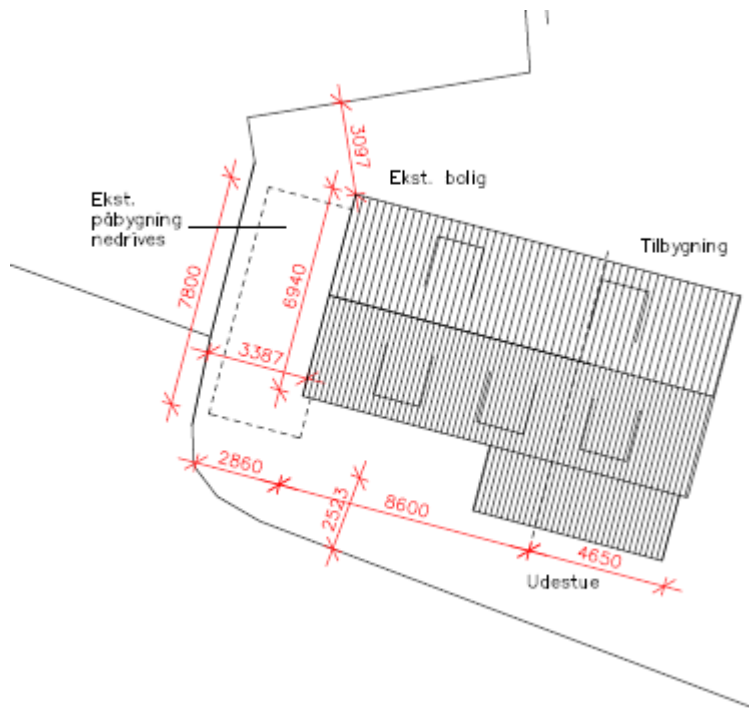
Figur 4: Situationsplan for den fremtidige bolig
