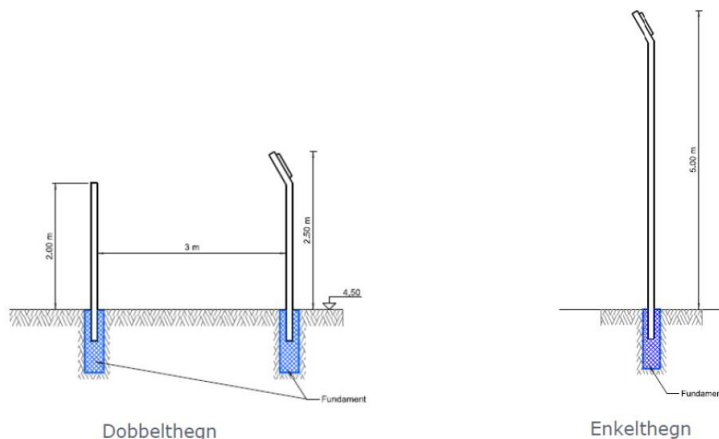
Figur 3 – Snittegning af hhv. dobbelthehn og enkelthehn
