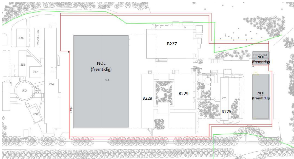
Figur 2 – Oversigtskort med placering af sikrings- og sikkerhedshegn (rød markering). Grønne linjer angiver strandbeskyttelseslinjen.
