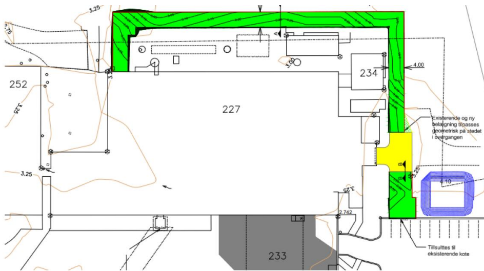
Figur 5 – Placering af ny vej – grøn markering.
