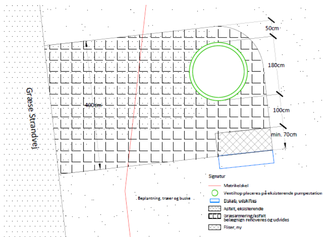
Fig. 3. Tilsendt fra ansøger. Situationsplan med mål for renoveringen af pumpestationen. Den nuværende asfaltering er indtegnet, samt markering af flisebelægning.
