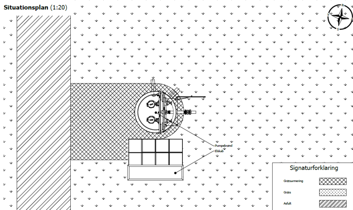
Fig. 2. Tilsendt fra ansøger. Situationsplan af renoveringen af pumpestationen.
