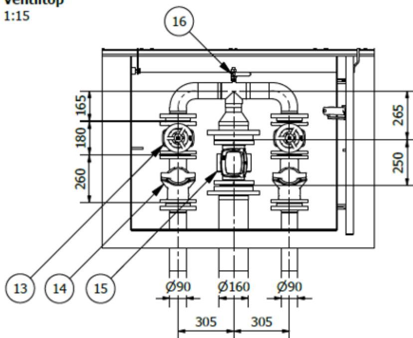
Fig. 5. Tilsendt fra ansøger. Tegning af pumpestationens ventiltop.
