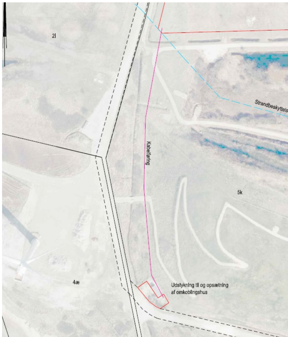
Figur 5, føringsvej for kabelnedlægning, fra ansøgningen
