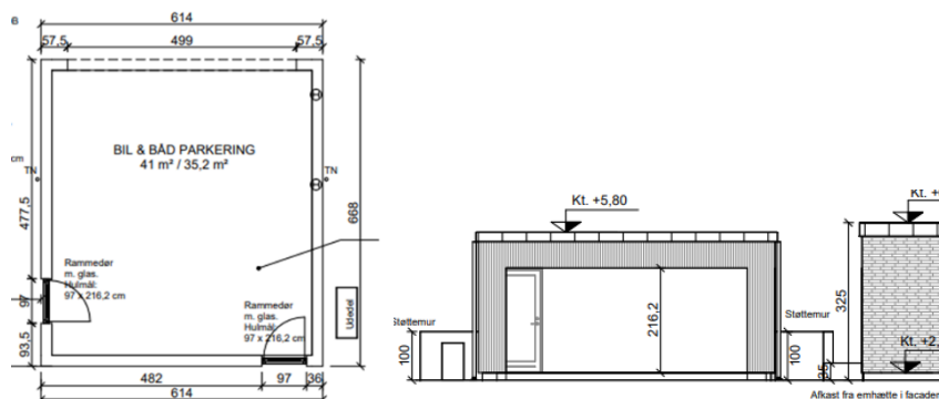
Grundplancarport/ skur
