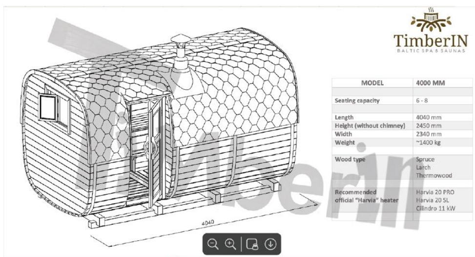
Fig. 4. Tilsendt fra ansøger. På figuren ses en illustration af den ansøgte sauna.
