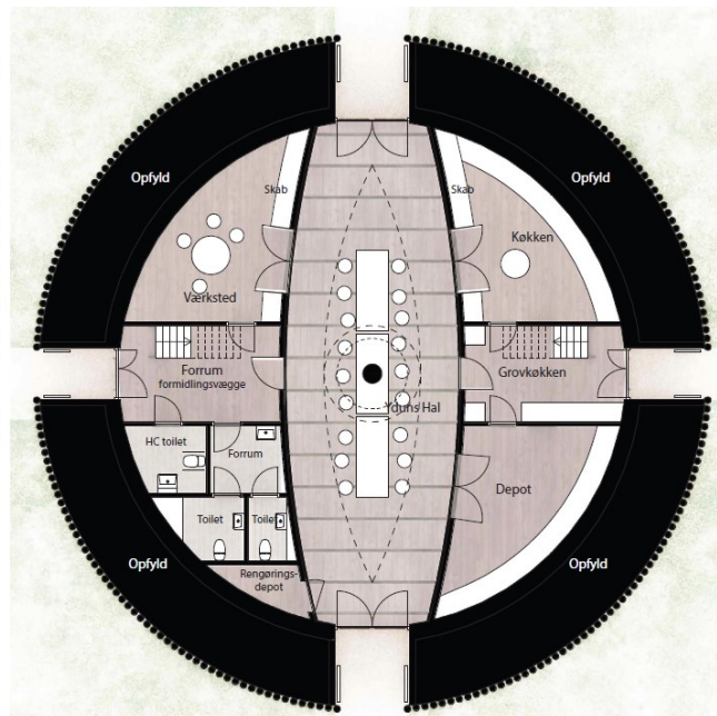
Figur 8, planløsning med arealer, fra ansøgningen.
