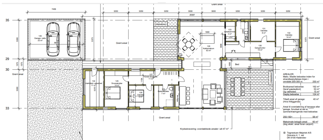
Grundplan ny bolig / under placering på grunden
