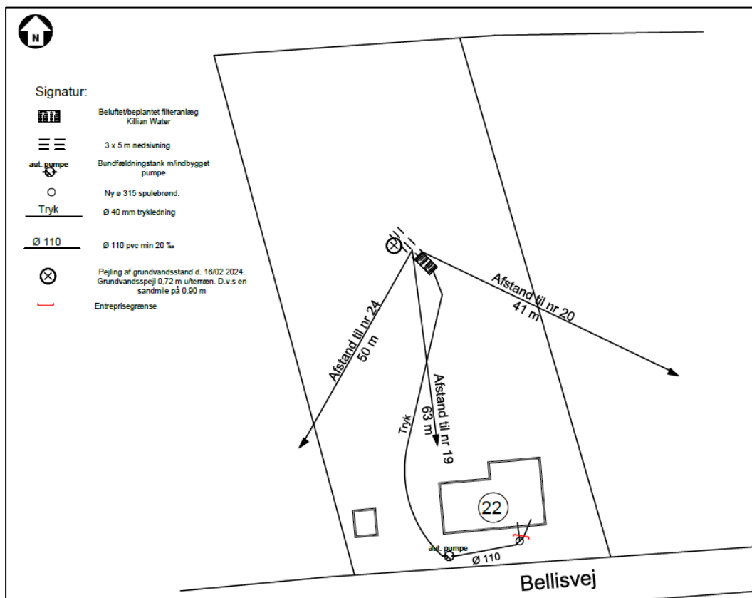
Situationsplan viser anlæggets placering på ejendommen.
