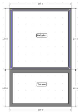
Tegning nyt badehus
