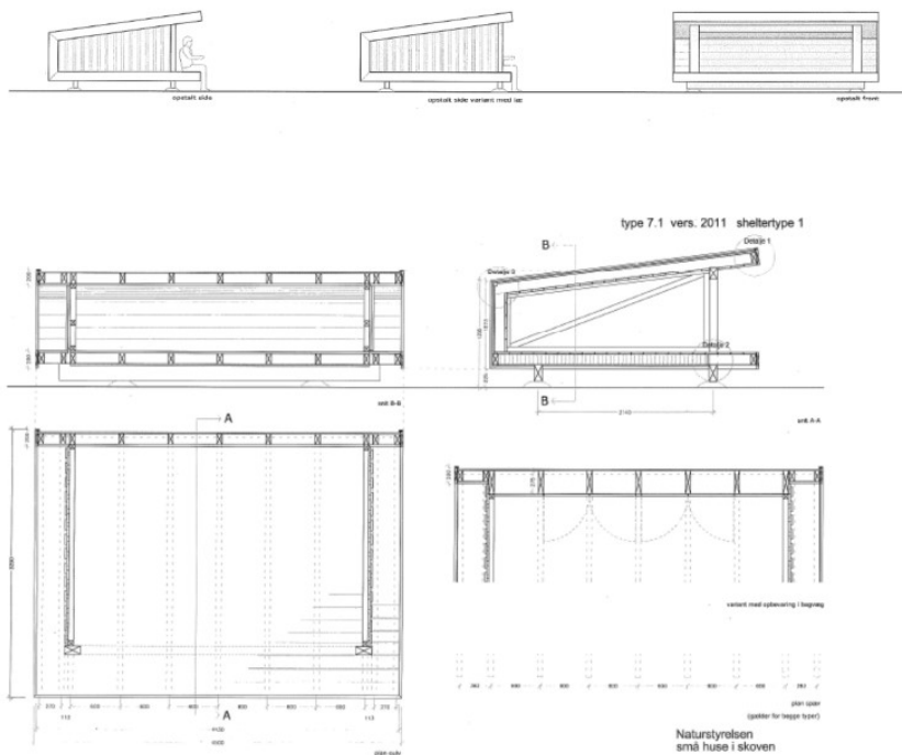
Figur 4, fra ansøgning, tegninger af shelter
