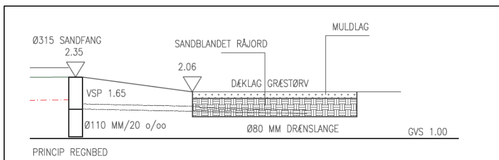
Principskitse
