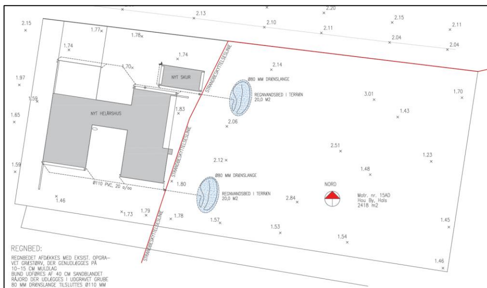
Plan viser placering af bedene
