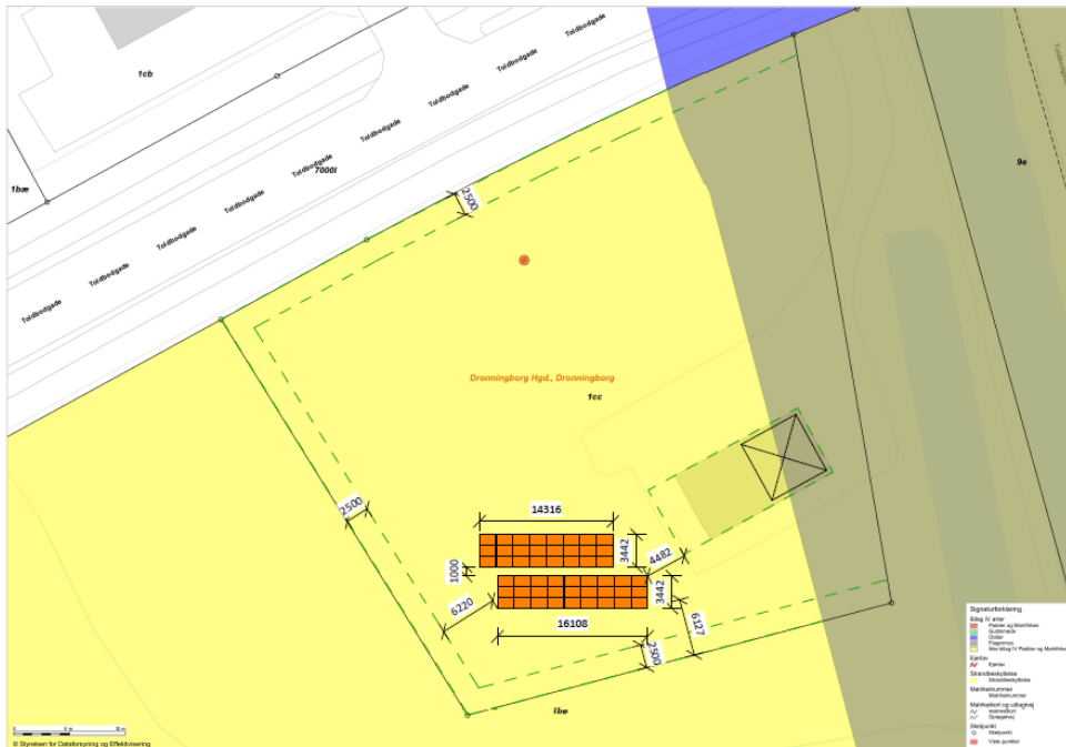
Situationsplan for anlægget
