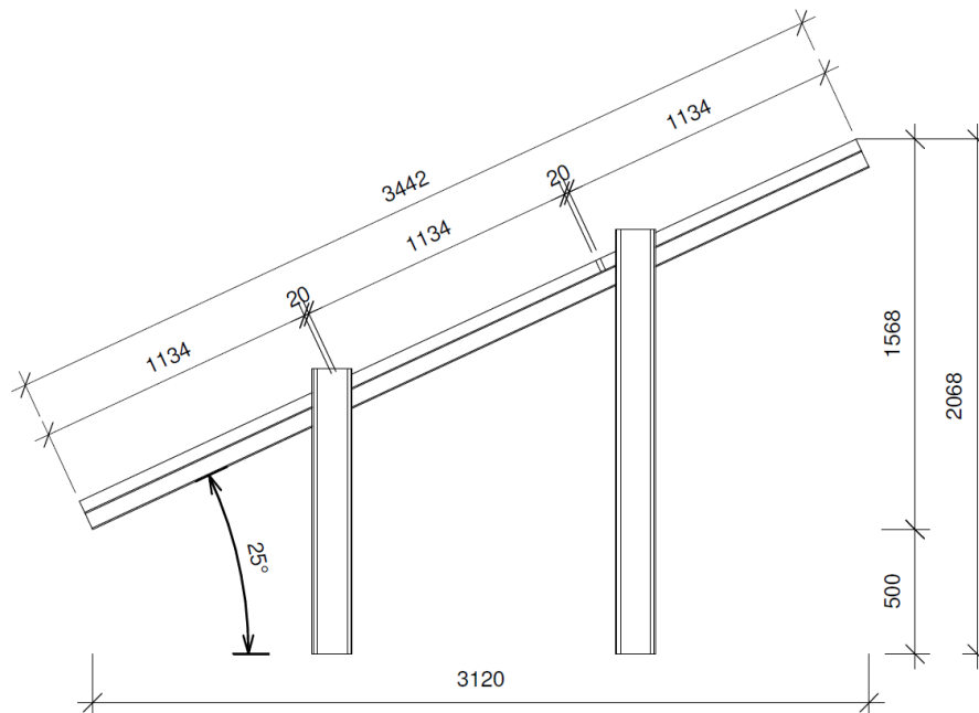
Tværsnit af anlægget
