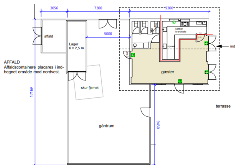
Fig. 3. Plantegning over det ansøgte indsendt af ansøger.
