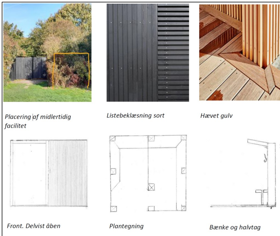
Figur viser tegning placering og detaljer for omklædningsfaciliteten.
