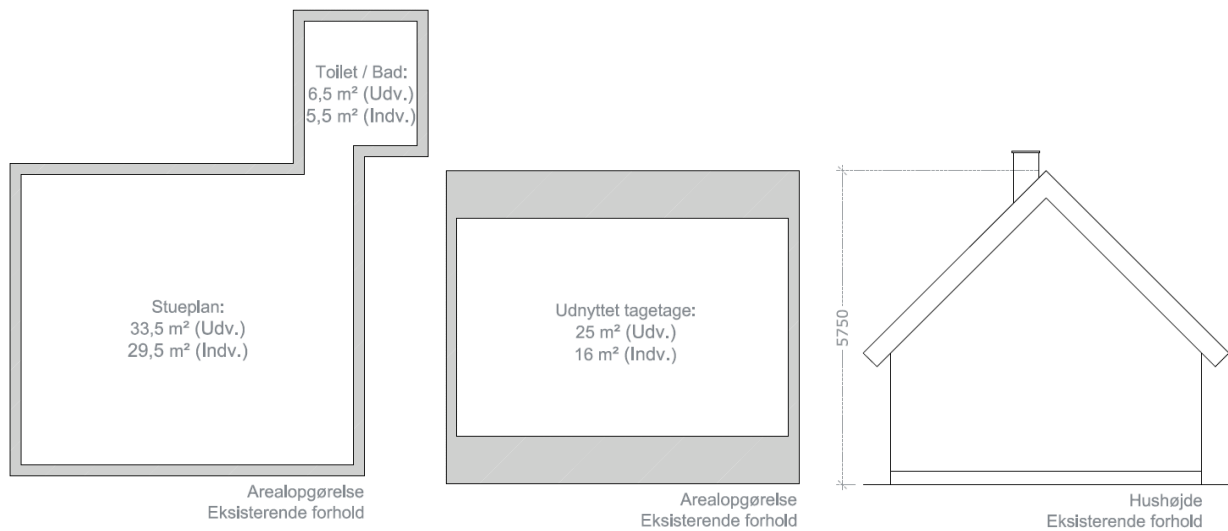
Figur 2. Grundplaner, arealopgørelse samt højde af det eksisterende sommerhus.
