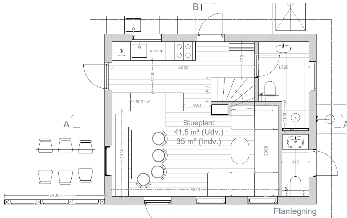
Plantegning af stueetagen
