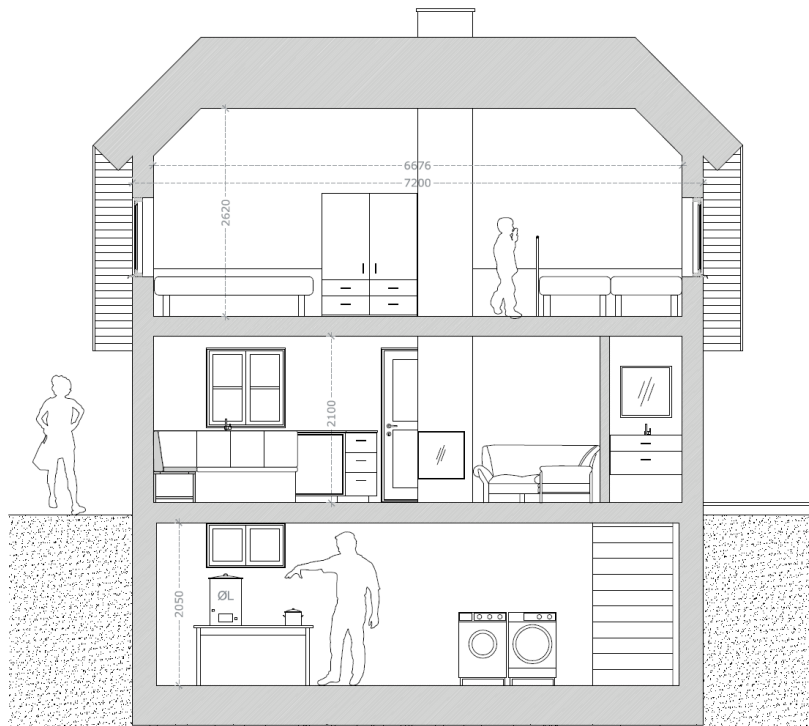
Tværsnit af det ansøgte sommerhus
