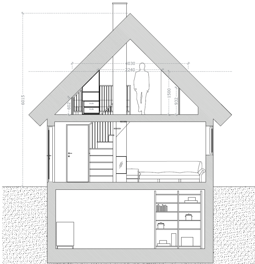
Tværsnit af det ansøgte sommerhus
