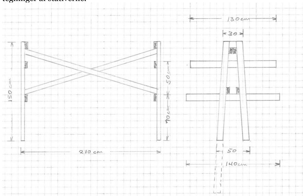
Fig. 3. Foto fra ansøgningen. Tegning af kajakstativ.
