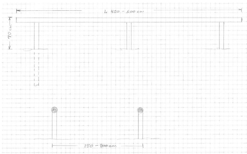
Fig. 4. Foto fra ansøgningen. Tegning af bådstativ.
