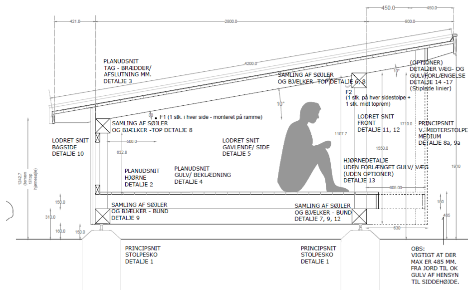
Figur 3. Tegning fra ansøgningen af den ansøgte sheltertype.
