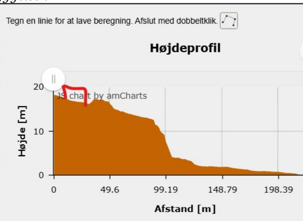
Højdeprofil fra udhus (vist rød) ned til kysten
