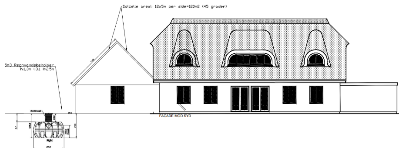
Placering i forhold til bebyggelsen
