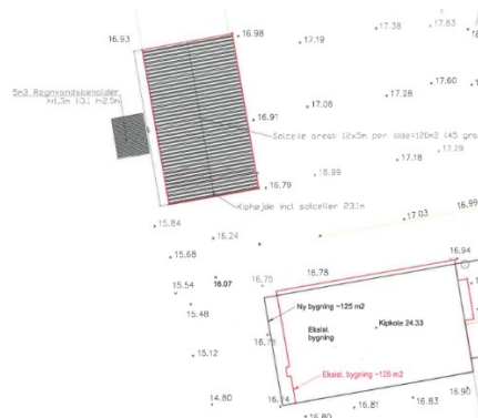
Situationsplan med regnvandsbeholder
