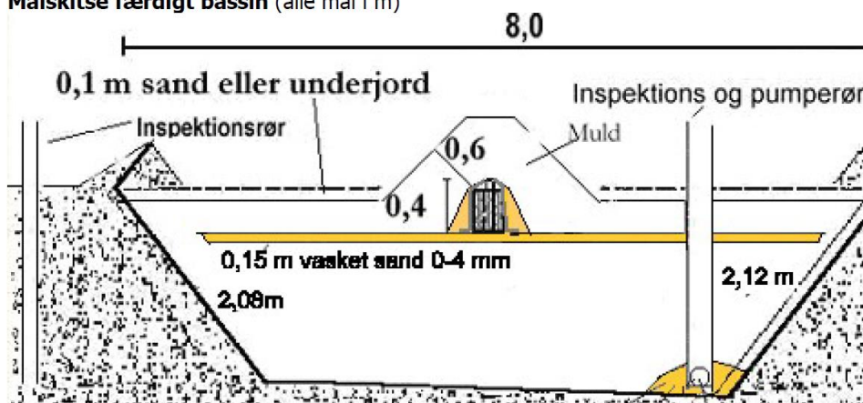
Fig. 2. Skitse over opbygning af bassinet
