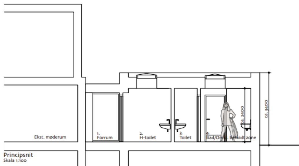
Fig. 7. Tilsendt fra ansøger. På figuren ses et principsnit af den ansøgte tilbygning.
