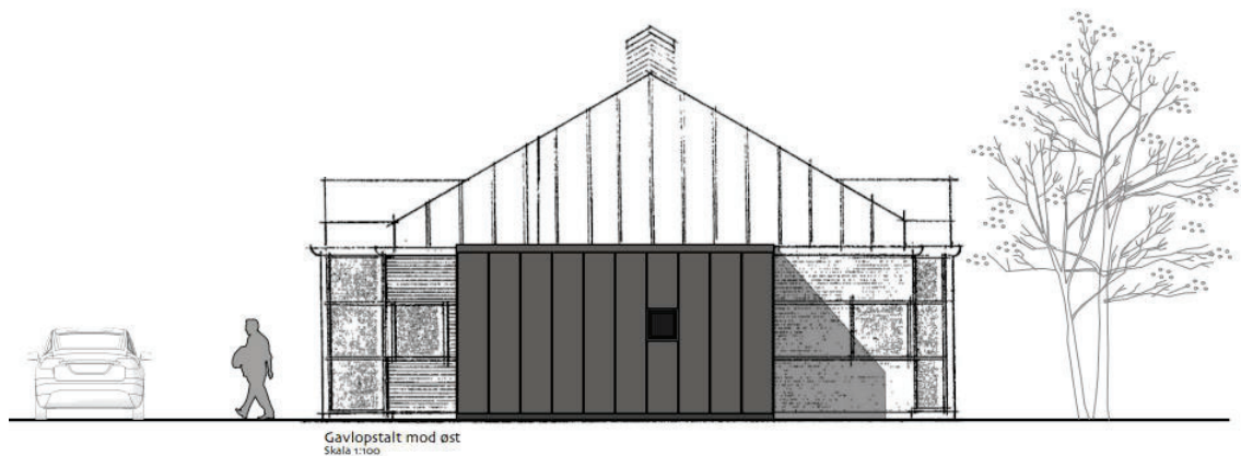
Fig. 6. Tilsendt fra ansøger. På figuren ses en tegning af den østvendte facade.
