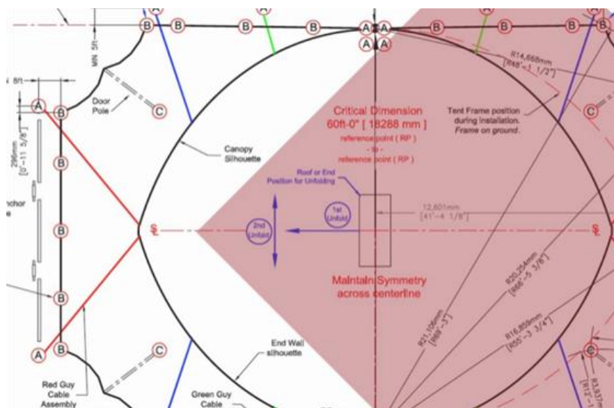
Fig. 3. Teknisk tegning af operateltet, som ønskes opstillet til arrangementet.
