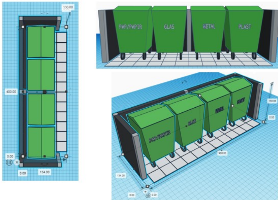
Fig. 1. Skitse af de forventede dimensioner af den ansøgte affaldsstation. Fra ansøgningsmaterialet.
