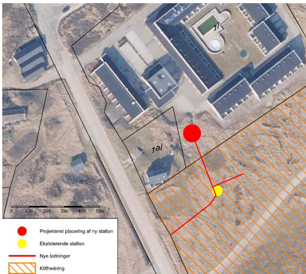
Oversigtskort over den eksisterende station, den nye station, og de nye ledninger der tilkobles til de eksisterende.
