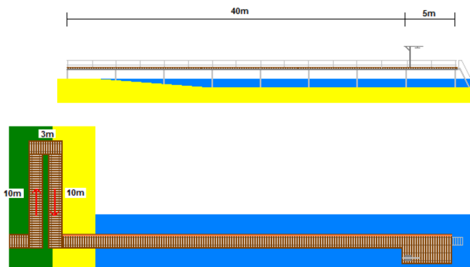
Fig. 1. Principskitse af anlægget fra ansøgningen
