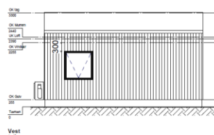
Facader for nyt sommerhus – syd og vest. Mod kysten (syd) ses til venstre
