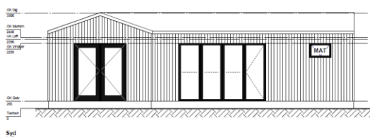
Facader for nyt sommerhus – syd og vest. Mod kysten (syd) ses til venstre
