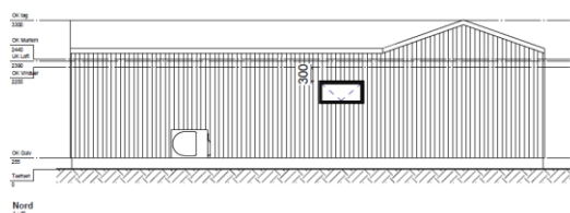
Facader for nyt sommerhus – nord og øst.
