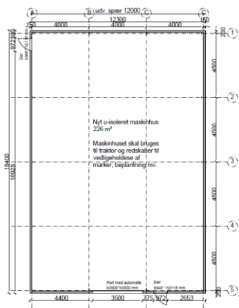
Grundplan
