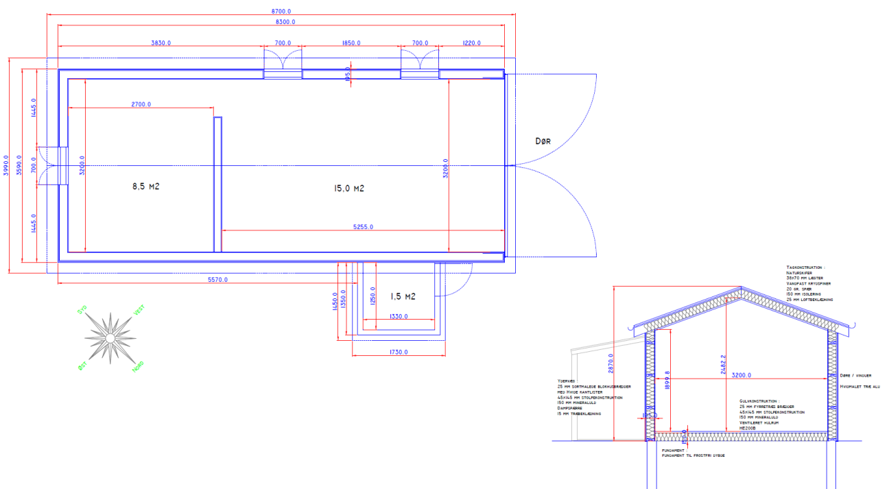
Figur 6. Grundplan- og snittegning af den ønskede bygning, indsendt i forbindelse med ansøgningen.
