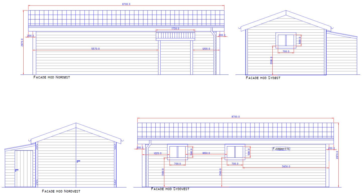
Figur 5. Facadetegninger af den ønskede bygning, indsendt i forbindelse med ansøgningen.
