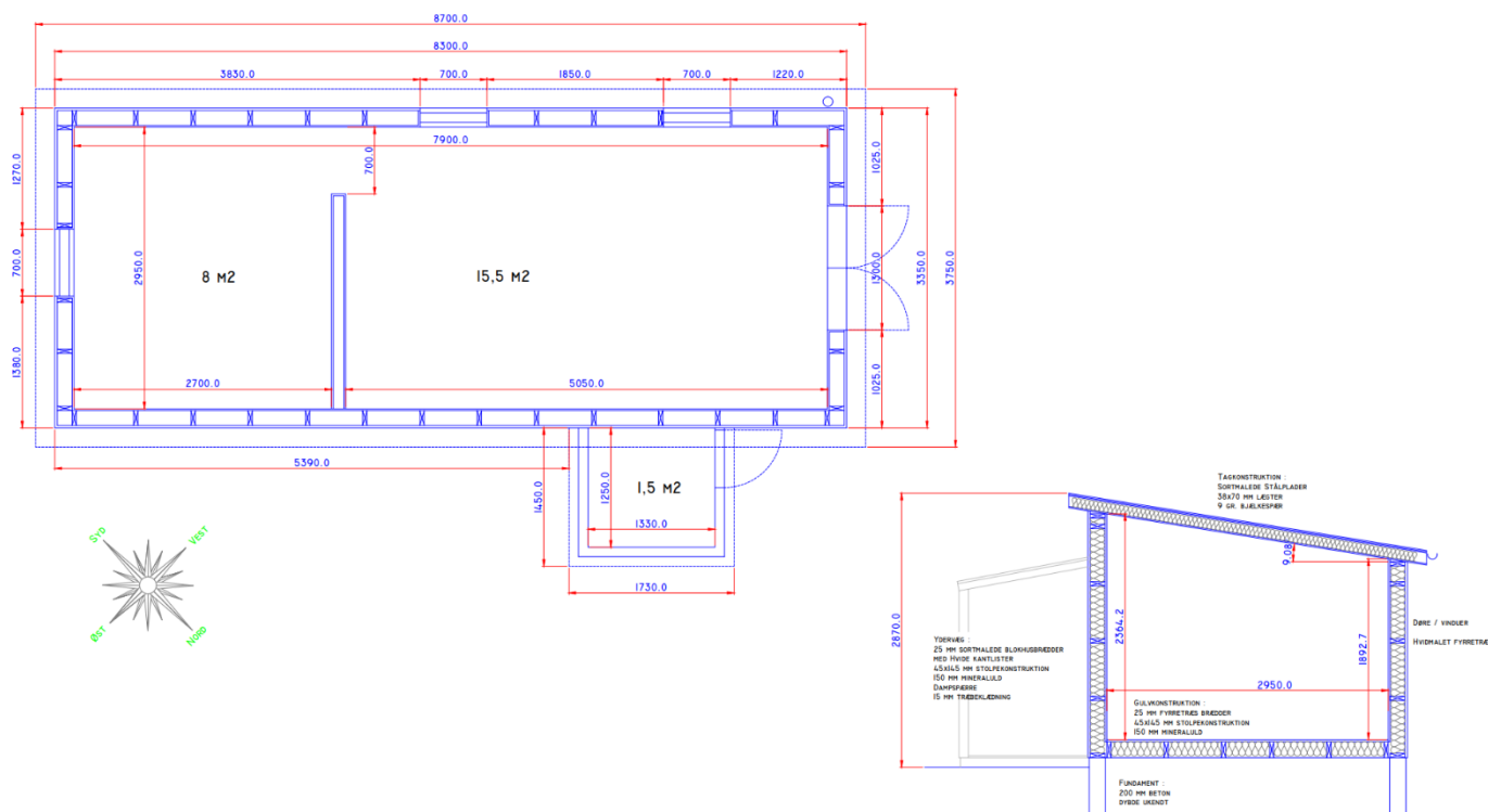
Figur 4. Grundplan- og snittegning af den nuværende bygning, indsendt i forbindelse med ansøgningen.
