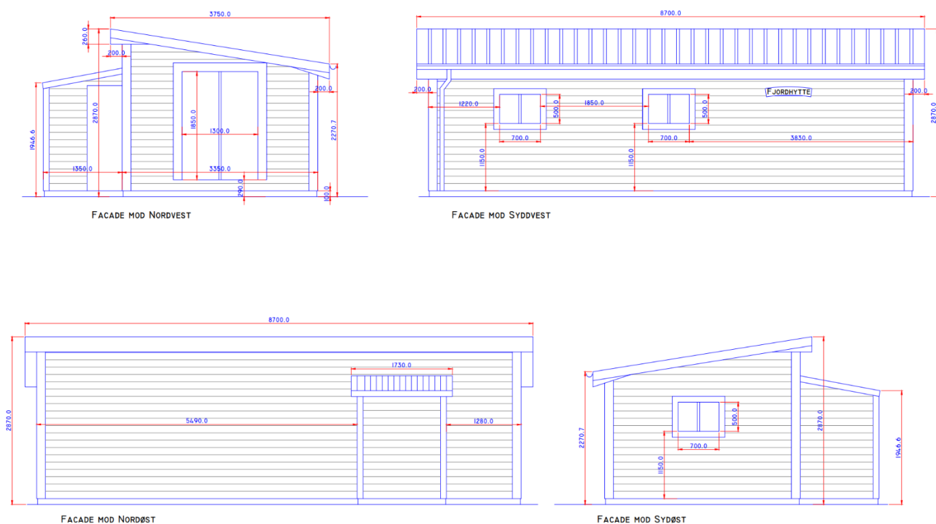
Figur 3. Facadetegninger indsendt i forbindelse med ansøgningen af den nuværende bygning.
