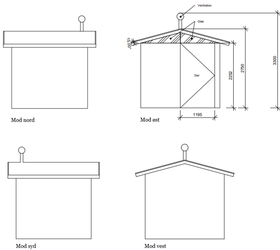
Fig. 4. Tegninger af det ansøgte muldtoilet indsendt af kommunen.
