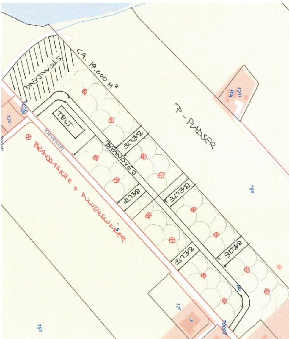
Situationsplan for arrangementet. Indsat fra ansøgningen.
