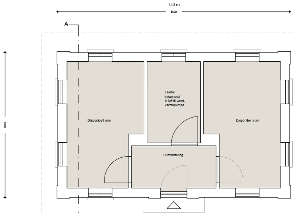
Grundplan nyt udhus
